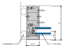
⑨ JAMB 6" = 1'-0"
