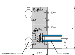
⑨ JAMB 6" = 1'-0"
