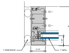
① JAMB 6" = 1'-0"
