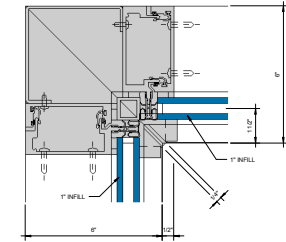
④ 90° INSIDE CORNER (SSG) G = 1'-0"
