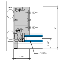
④ ALT. SSG JAMB Ø = 1'-0"
