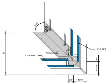
② 90° OUTSIDE CORNER (SSG) G = 1'-0"
