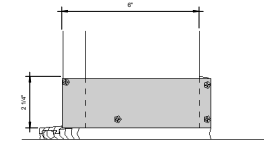
④ SILL END CAP @ DOOR JAMB 6" = 1'-0"
