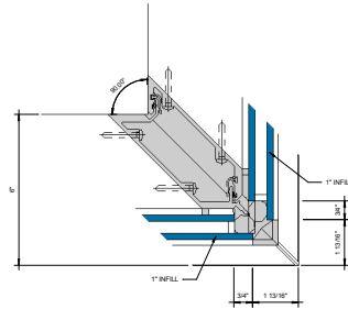
② 90° OUTSIDE CORNER (SSG) G = 1'-0"
