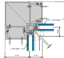
④ 90° INSIDE CORNER (SSG) G = 1'-0"
