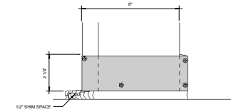
④ SILL END CAP @ DOOR JAMB 6" = 1'-0"
