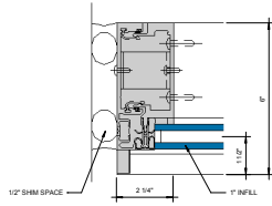
① JAMB 6" = 1'-0"
