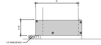
④ SILL END CAP @ DOOR JAMB 6" = 1'-0"
