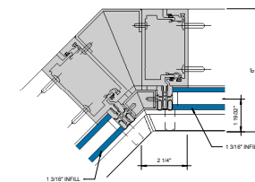
⑧ 135° INSIDE CORNER (SSG) G = 1'-0"
