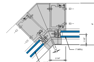
⑧ 135° INSIDE CORNER (SSG) G = 1'-0"
