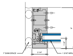
⑩ JAMB 6" = 1'-0"
