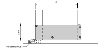
④ SILL END CAP @ DOOR JAMB 6" = 1'-0"
