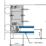
3 ALT. SSG JAMB 6" = 1'-0"
