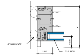
④ ALT. SSG JAMB Ø = 1'-0"
